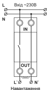
Схема підключення
